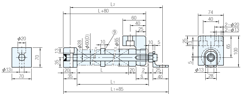
2 條彈簧構造圖
